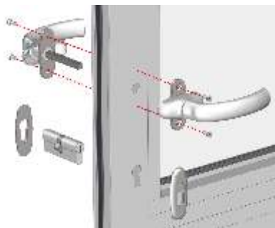
Poignées avec rosaces et canon de sécurité
