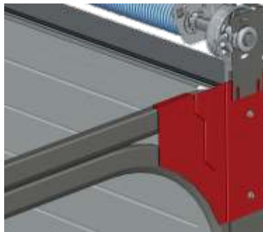
Renfort d'angle sur courbe de renvoi
